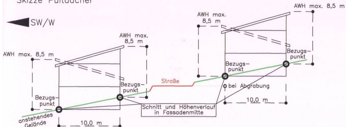
Skizze Pultdächer
